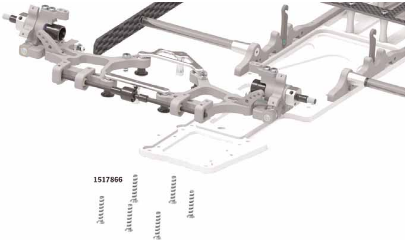
Querlenker hinten oben und Getriebeplatte/A-arm rear upper and transmission bracket
